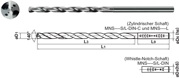
■ MNS○○○○L-OC-, MNS○○○○L-OCDC-Typ
