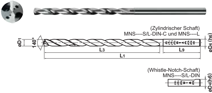
■ MNS○○○○-L○C-, MNS○○○○-L○C-C-Typ
