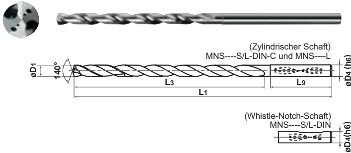
■ MNS○○○○-L○C-, MNS○○○○-L○C-Typ
