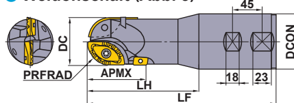
● Weldonschaft (Abb. 3)
