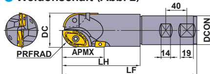
● Weldonschaft (Abb. 2)
