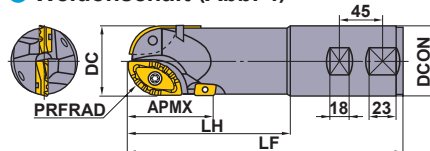
● Weldonschaft (Abb. 4)
