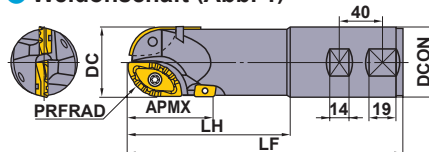
● Weldonschaft (Abb. 1)
