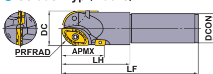
● Gerader Typ (Abb. 8)
